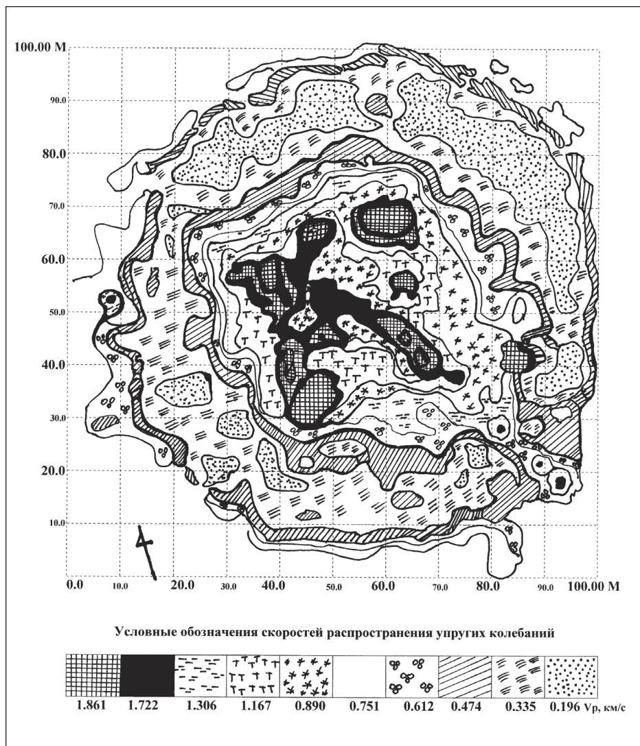
Рис. 1. Горизонтальный профиль сопки Шум-гора на отметке +1 м от горизонта.
