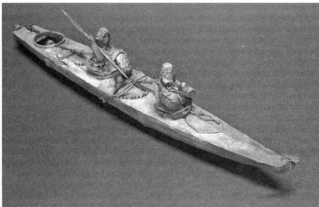
Рис. 1. Модель трехлючного алеутского женского каяка с Лисьих островов (№ 615) 1 . Начало XIX в. Дерево, пузырь сивуча, жилы. Привезена капитан-лейтенантом Ю.Ф. Лисянским из первого российского кругосветного плавания (1803–1806 гг.).
